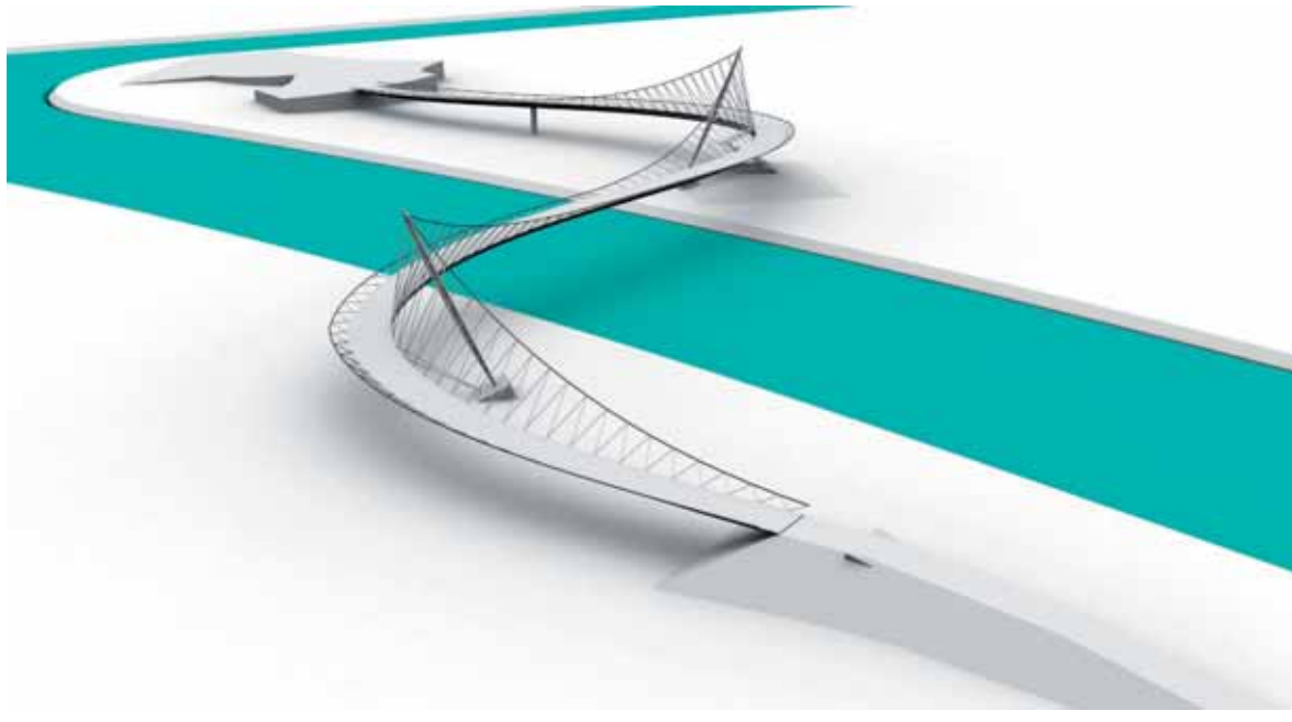
Collegebrug te Kortrijk / Computertekening: Ney & Partners
