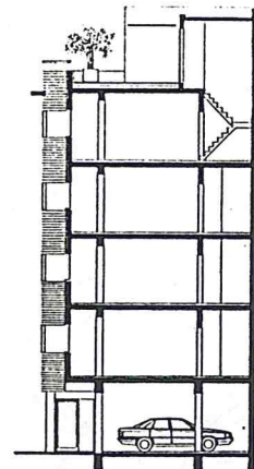
Dwarsdoorsnede.
